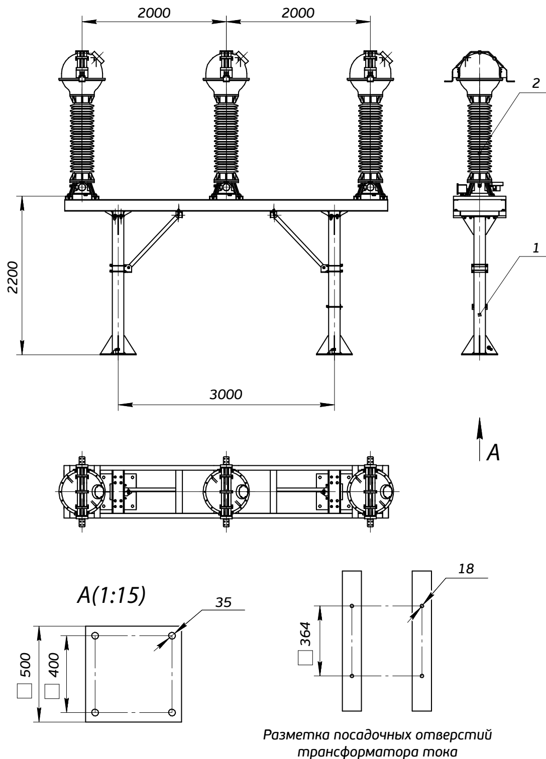
Габаритные, установочные и присоединительные размеры опорной стойки металлоконструкции на 3 трансформатора тока ТГ-СВЭЛ-110
